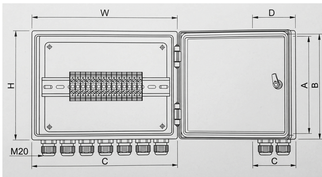
Клеммная коробка: зажимы, вводы
